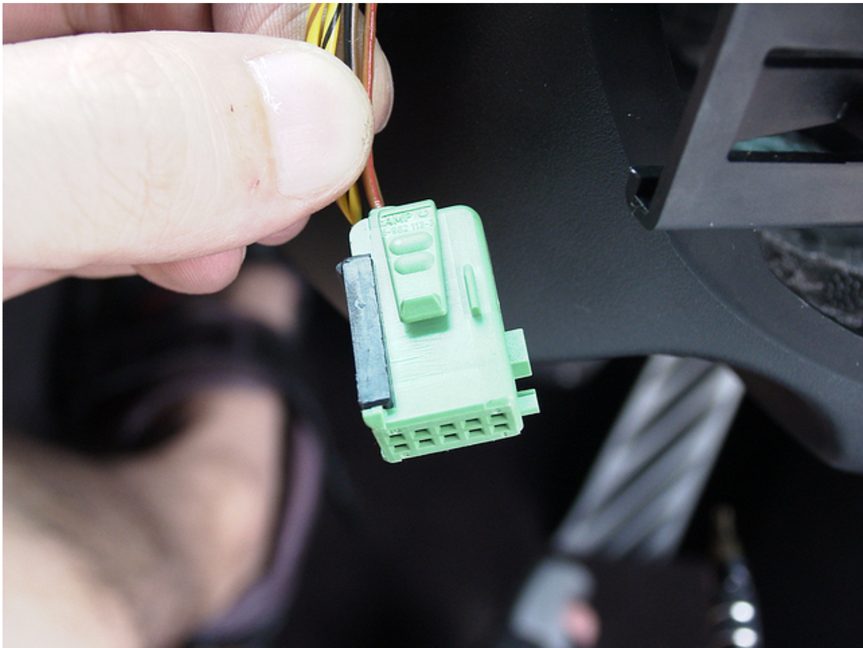
車両本体からコンタクトリングへのコネクタ（10ピン）
